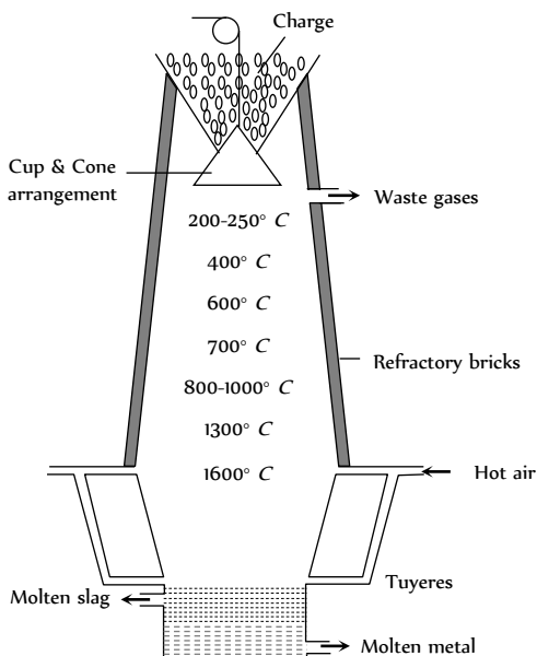
Fig. 16.5. Blast Furnace
